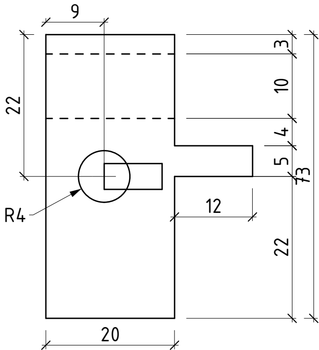
WIDOK Z PRZODU SKALA 1:6
