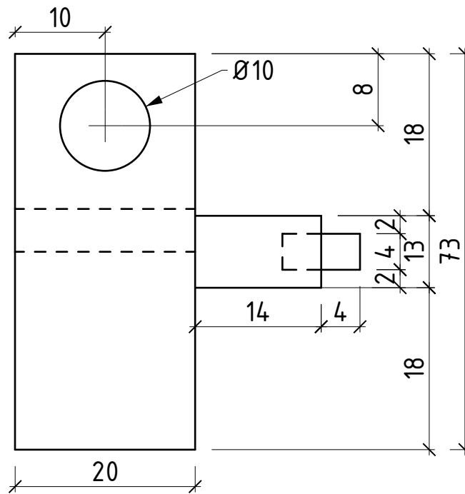
RZUT Z GÓRY SKALA 1:6
